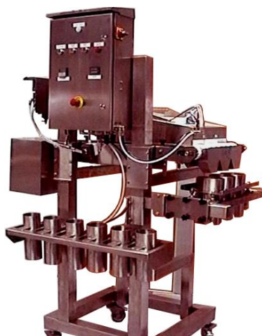
Distributeur de fromage râpé sur operculeuse
