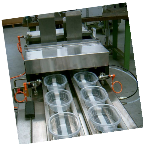
Dépileur 2 pistes
