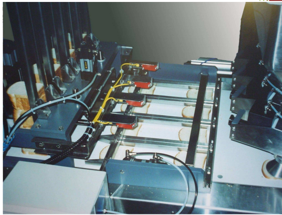
Alimentation automatique du dépileur en barquettes PSE
