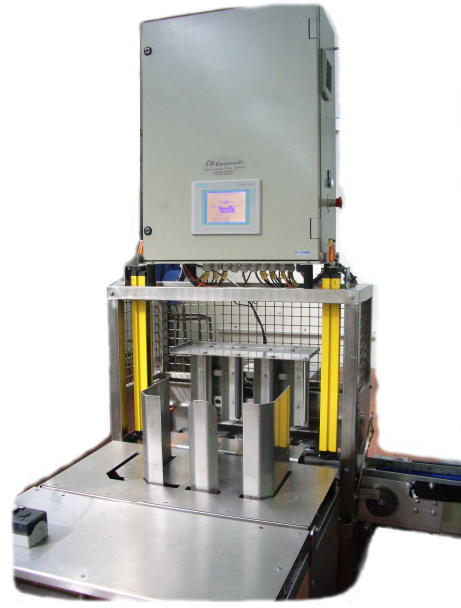
Empileur
