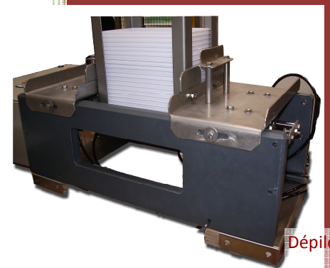
Dépilage de seaux avec alimentation automatique
