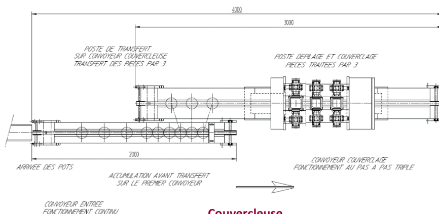
Couvercleuse Schéma de principe
